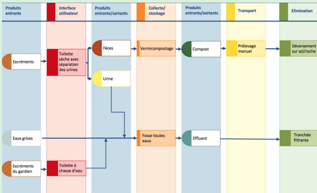
Schéma du traitement des résidus à la cabane Schönbühl
